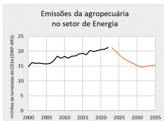
Figura 14 - Histórico (2000 a 2022) e projeção (2023 a 2035) das emissões da agropecuária dentro do setor de Energia
