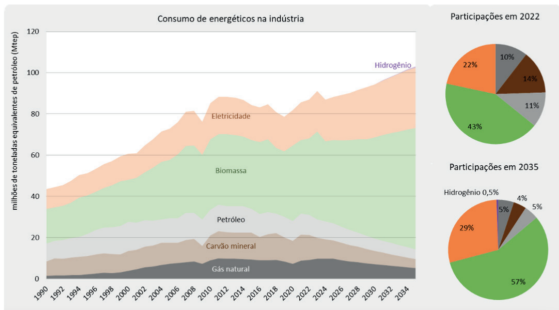
Figura 6 - Histórico (1990 a 2022) e projeção (2023 a 2035) do consumo de energéticos na indústria, destacando eletricidade, hidrogênio e as fontes primárias dos combustíveis utilizados
