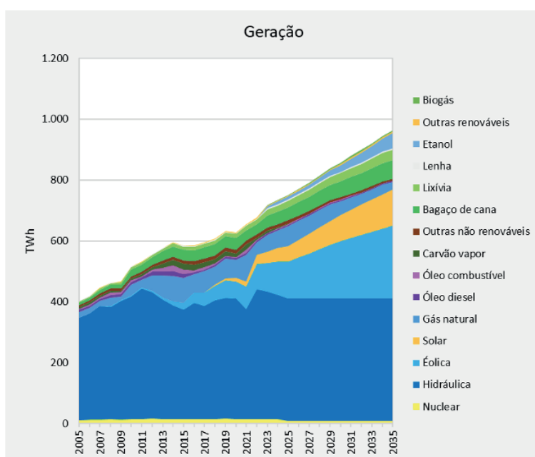
Figura 10 - Histórico (2005 a 2022) e projeção (2023 a 2035) da geração de energia elétrica por fonte
