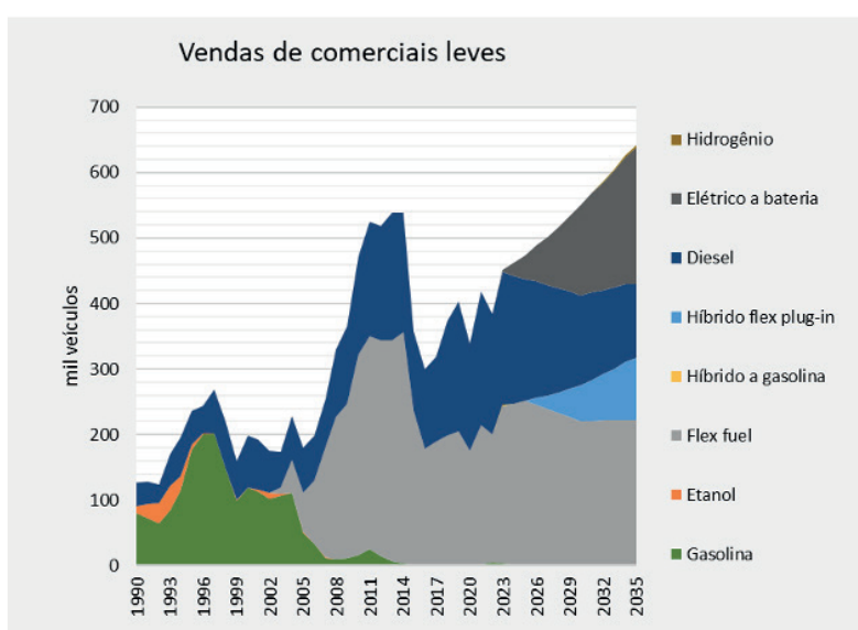
Figura 4 - Histórico (1990 a 2022) e projeção (2023 a 2035) das vendas anuais de novos veículos comerciais leves segundo tecnologias de propulsão
