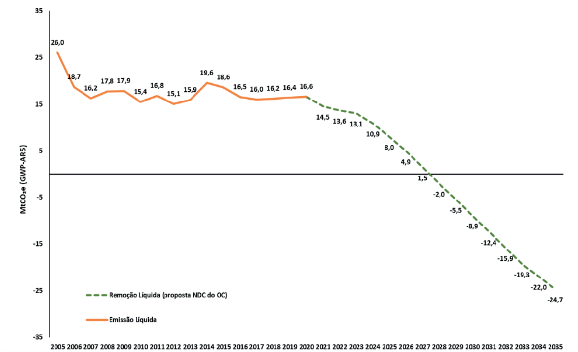
Figura 23 - Trajetória tendencial e da proposta da NDC das emissões líquidas de SPD entre 2020 e 2035.
