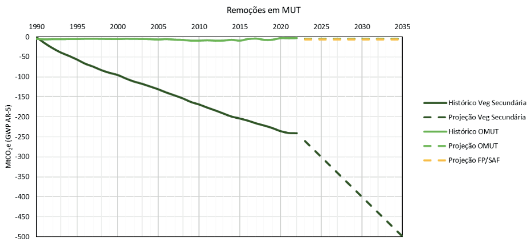
Figura 27 - Histórico e projeções de remoções relacionadas ao crescimento de vegetação secundária, à implementação de florestas plantadas (FP) e sistemas agroflorestais (SAF) e a outras mudanças de uso da terra (OMUT). As metas relacionadas à implementação de novas florestas plantadas e sistemas agroflorestais são aditivas a partir de 2022 e, por isso, não possuem curva do histórico.
