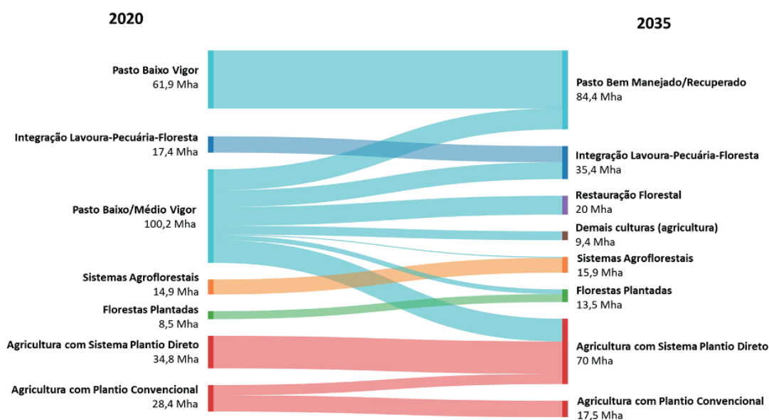
Figura 24 - Conversões de uso e manejo do solo pelo setor de agropecuária entre 2020 e 2035.
