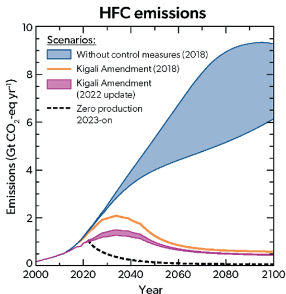
Figura 15 - Histórico (2000 a 2021) e projeção (2022 a 2050) das emissões, em milhões de toneladas de CO 2 e, referentes ao uso mundial de HCFs (OMM, 2022)
