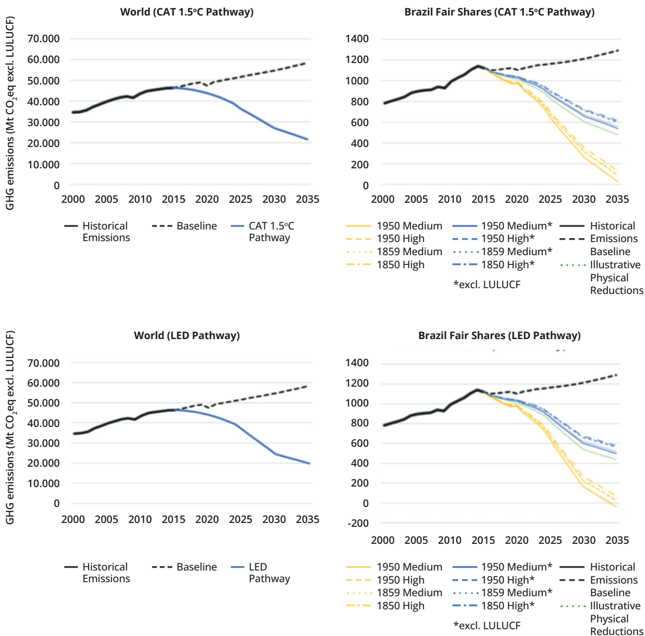
Figura 2 - Trajetórias globais de mitigação e os “fair shares” do Brasil (Fonte: Holz, 2024)
