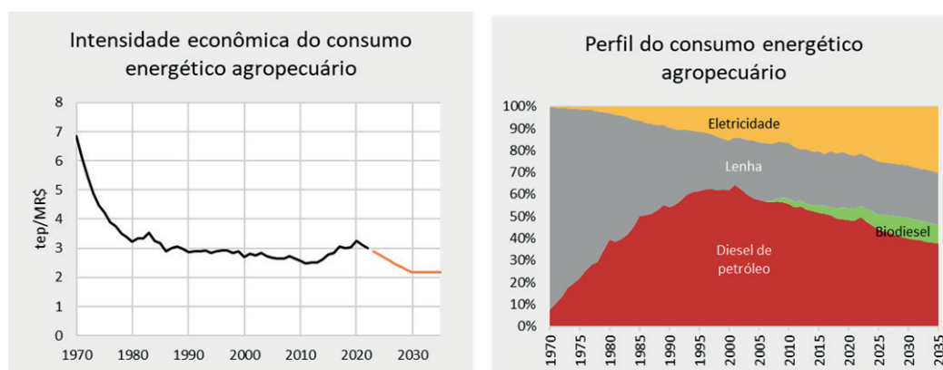
Figura 13 - Histórico (1970 a 2022) e projeção (2023 a 2035) da intensidade econômica do consumo energético agropecuário e histórico (1970 a 2022) e projeção (2023 a 2035) do perfil do consumo energético agropecuário (% baseada em tep)
