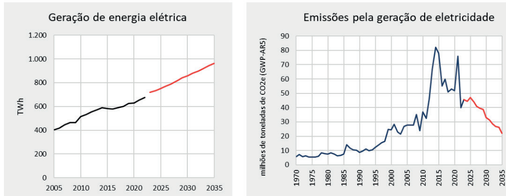
Figura 8 - Histórico (2005 a 2022) e projeção (2023 a 2035) da geração de energia elétrica e Histórico e projeção das emissões associadas, em milhões de toneladas de CO 2 e
