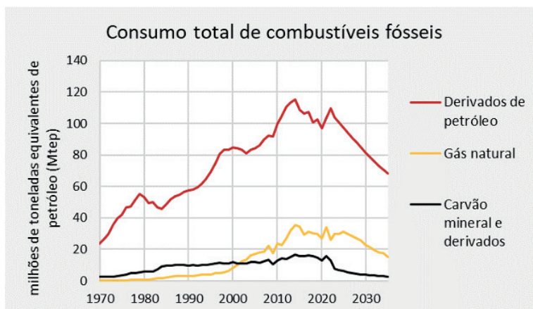
Figura 7 - Histórico (1970 a 2022) e projeção (2023 a 2035) do consumo total de petróleo, gás natural, carvão mineral e derivados
