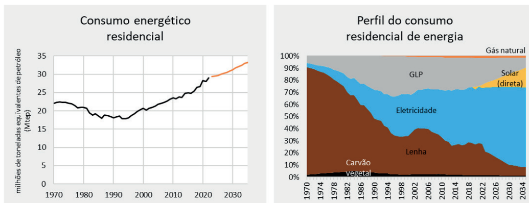
Figura 11 - Histórico (1970 a 2022) e projeção (2023 a 2035) do consumo energético residencial e histórico (1970 a 2022) e projeção do perfil do consumo energético residencial (% baseada em tep)
