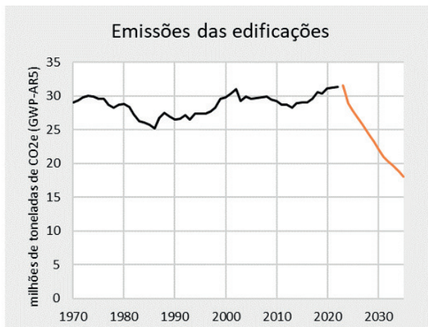
Figura 12 - Histórico (1970 a 2022) e projeção (2023 a 2035) das emissões das edificações
