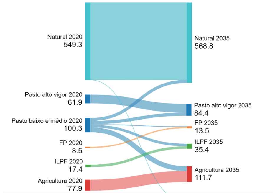
Figura 25 - Conversões da cobertura e uso da terra no território brasileiro, totalizando 8,5 milhões de hectares, considerando as metas dos setores de Agricultura e Mudanças de Uso da Terra e Florestas para 2035 e o ano-base de 2020.
