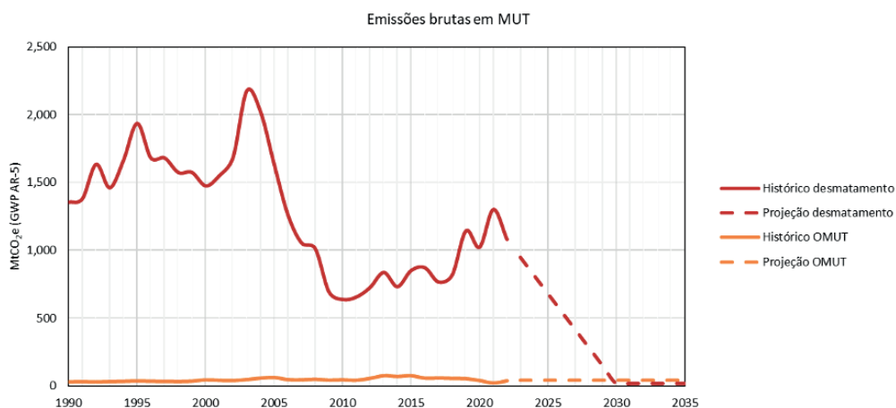
Figura 26 - Histórico e projeções de emissões brutas relacionadas ao desmatamento e a outras mudanças de uso da terra (OMUT).
